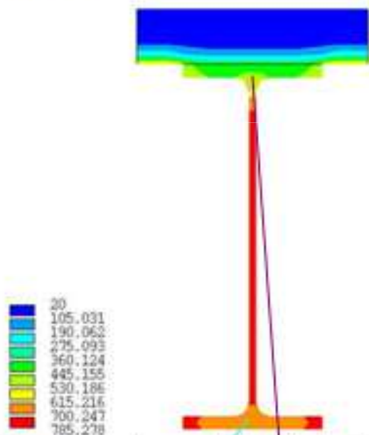
Exemple de champs de températures
