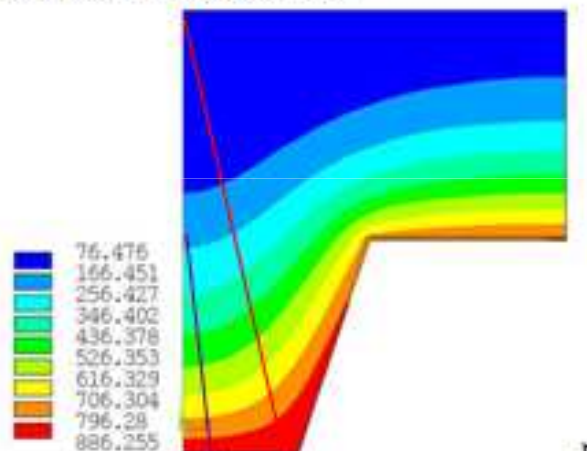
Bac acier et dalle béton
