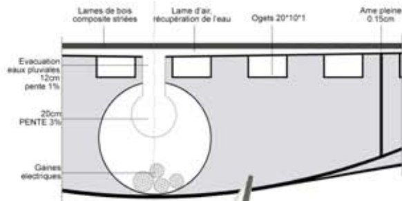
Détail structure sur tablier 1/50
