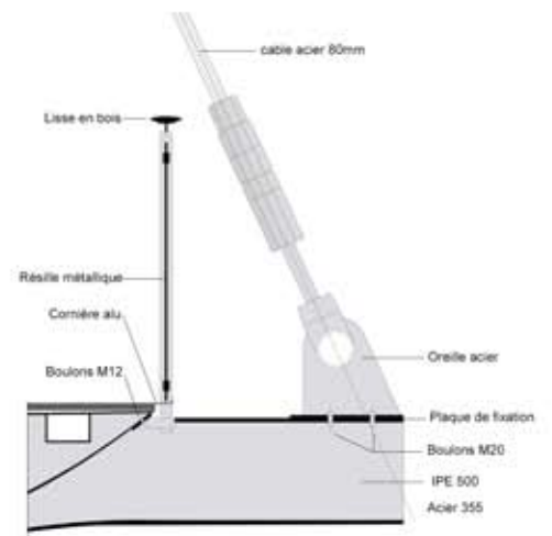
Détail structure d'accroche de hauban 1/50
