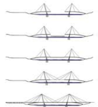
Cinématique de montage
